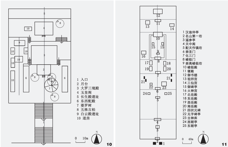
图10 阳台宫平面 Fig. 10 The plan of Yangtai Palace
